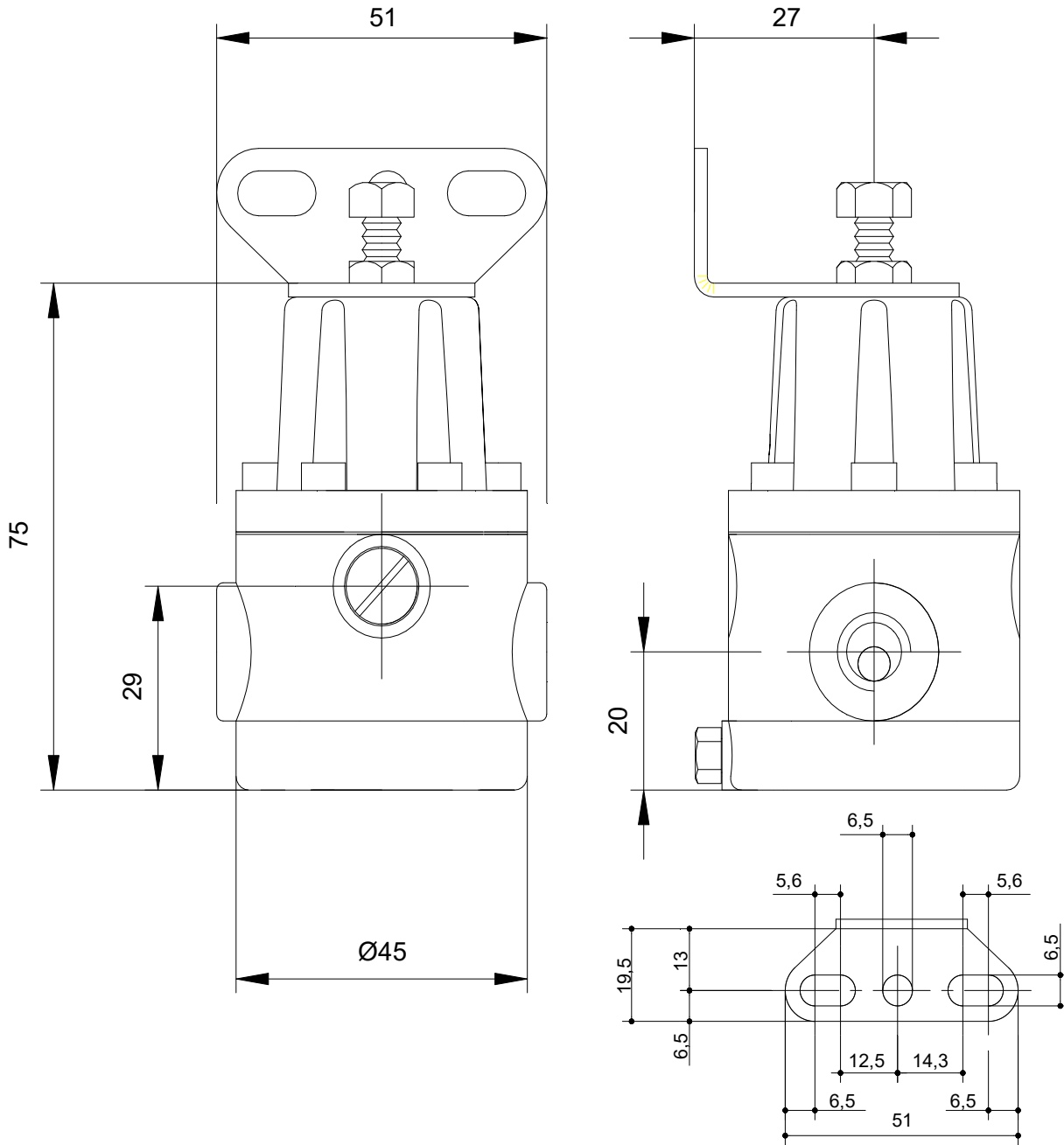
STAFFA ACCIAIO INOX BRACKET STAINLESS STEEL
